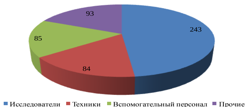
Рисунок 2 – Структура персонала, занятого исследованиями и разработками в Брянской области в 2020 году, человек
