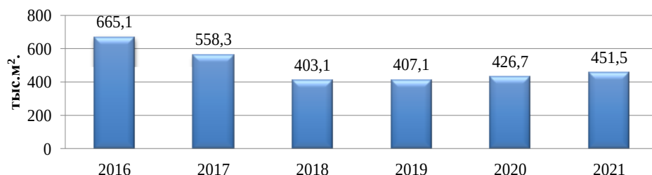
Рисунок 2 – Динамика ввода жилья на территории Брянской области в 2016-2021 гг., тыс.м².
