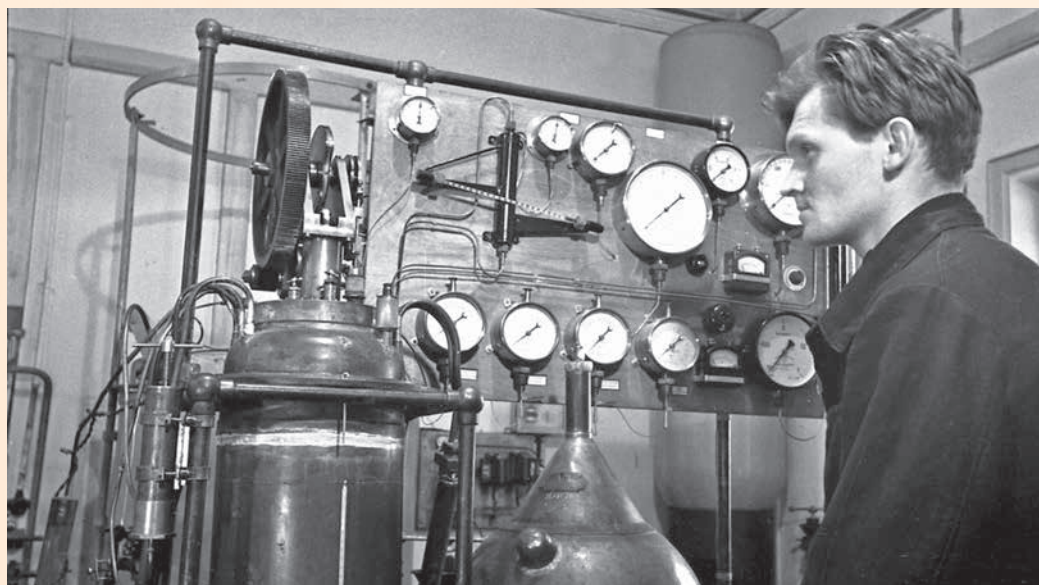
Сотрудник лаборатории Института физических проблем АН СССР около установки для получения жидкого гелия, 1940
