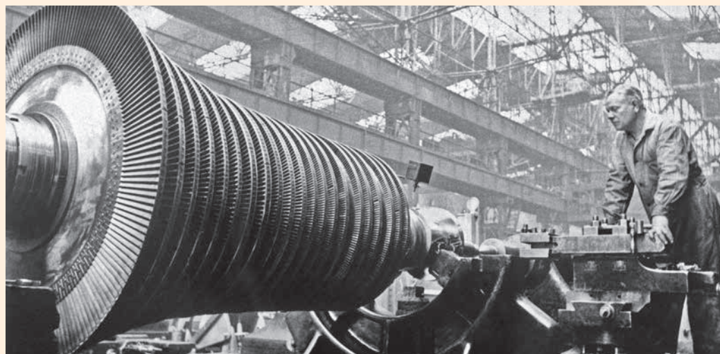
Обработка ротора паровой турбины на Ленинградском металлургическом заводе, 1941
